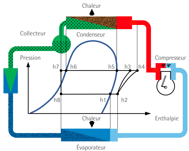
Exemple d'un circuit frigorifique.
